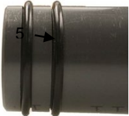
Abb. 29: Verlängerungsrohrende mit breiten O-Ringen - Schlauchanschluss
