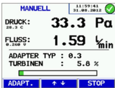
Abb. 51: Manueller Modus
